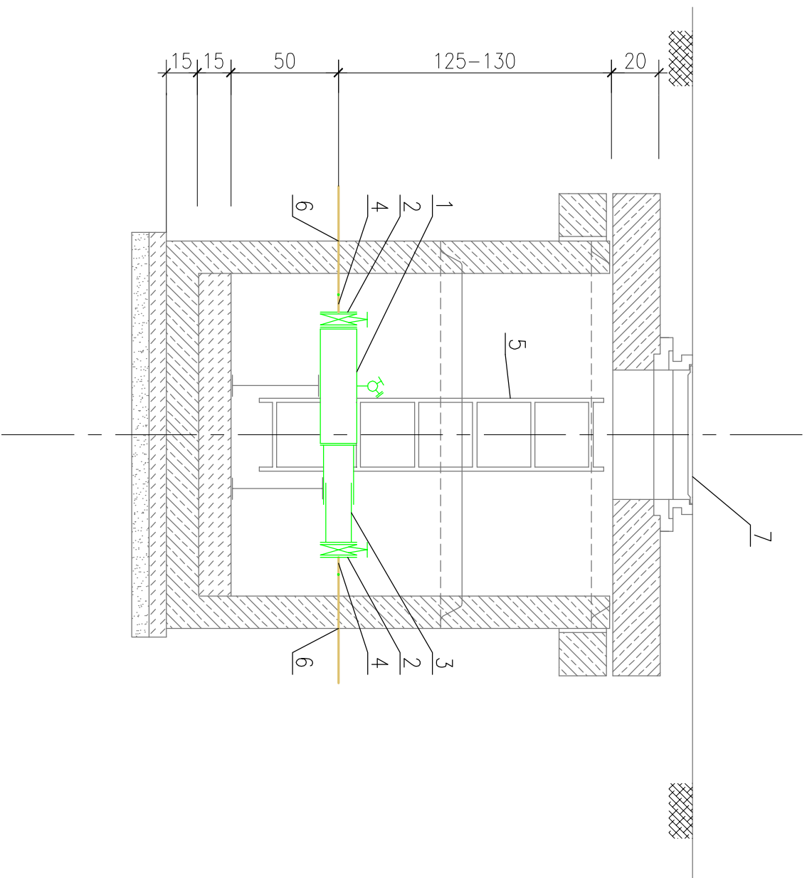
ZESTAWIENIE WYPOSAŻENIA STUDNI – ŚREDNICA D w =1500mm
